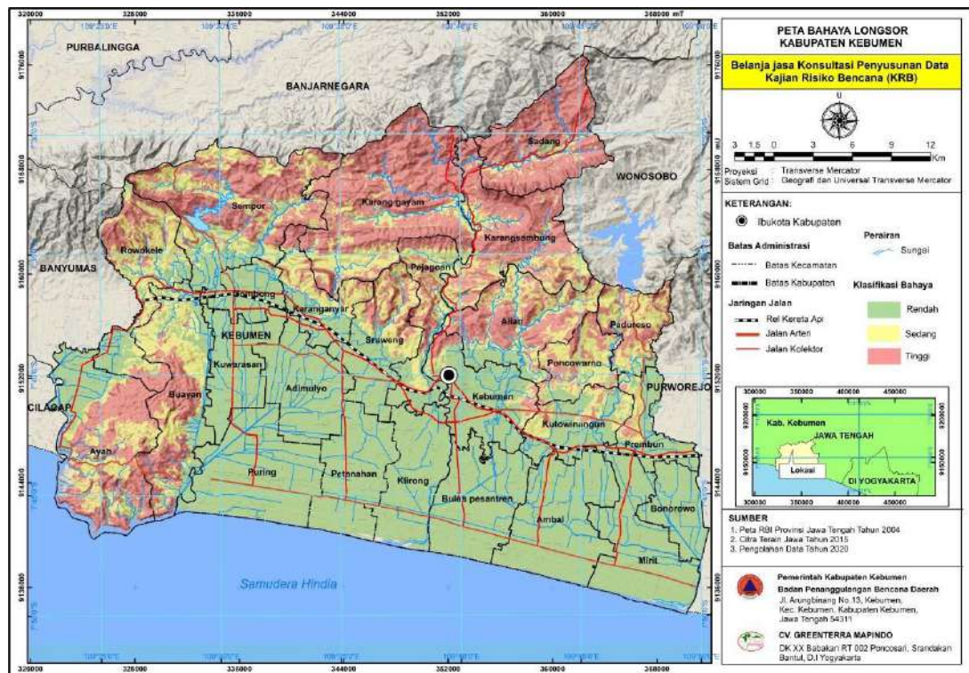
Gambar 2.8 Peta Bahaya Tanah Longsor Kabupaten Kebumen
