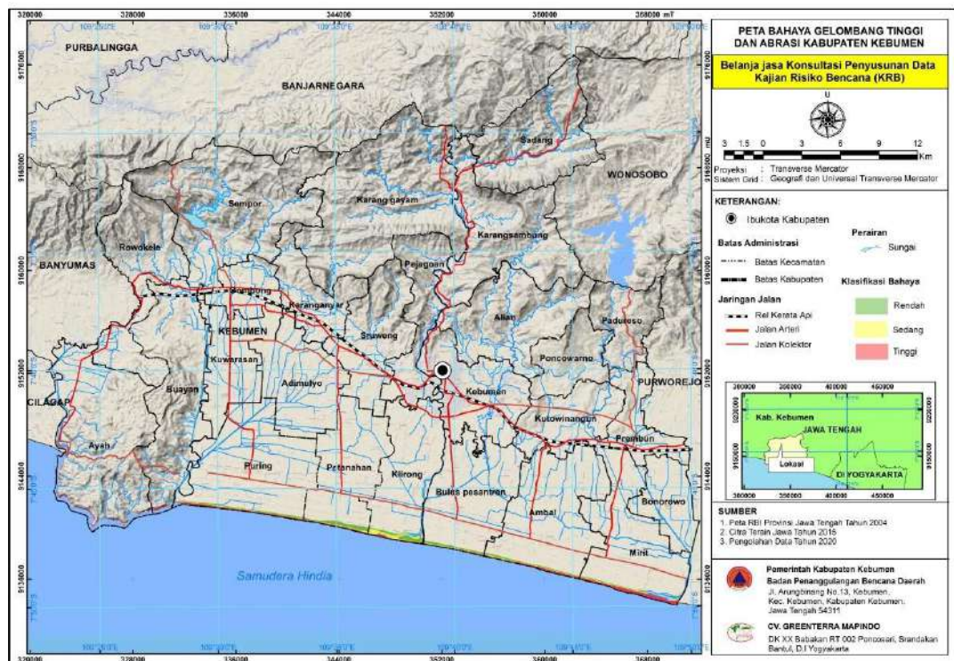
Gambar 2.14 Peta Bahaya Gelombang Ekstrem dan Abrasi Kabupaten Kebumen
