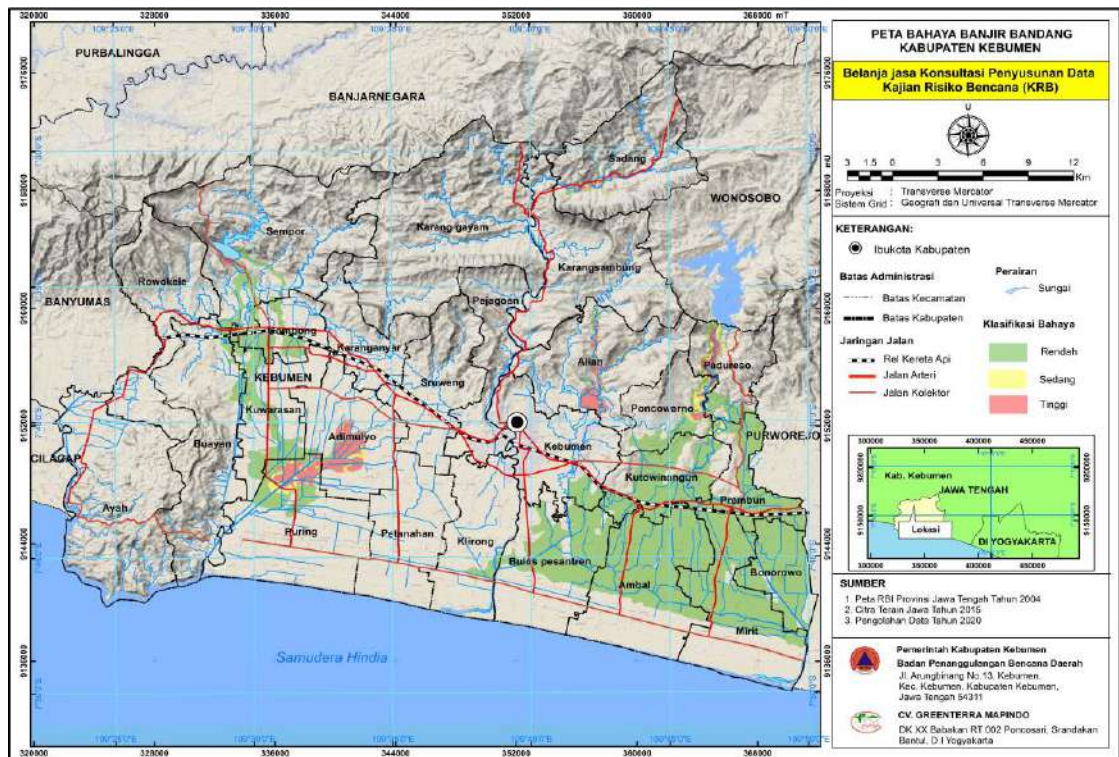
Gambar 2.7 Peta Bahaya Banjir Bandang Kabupaten Kebumen
