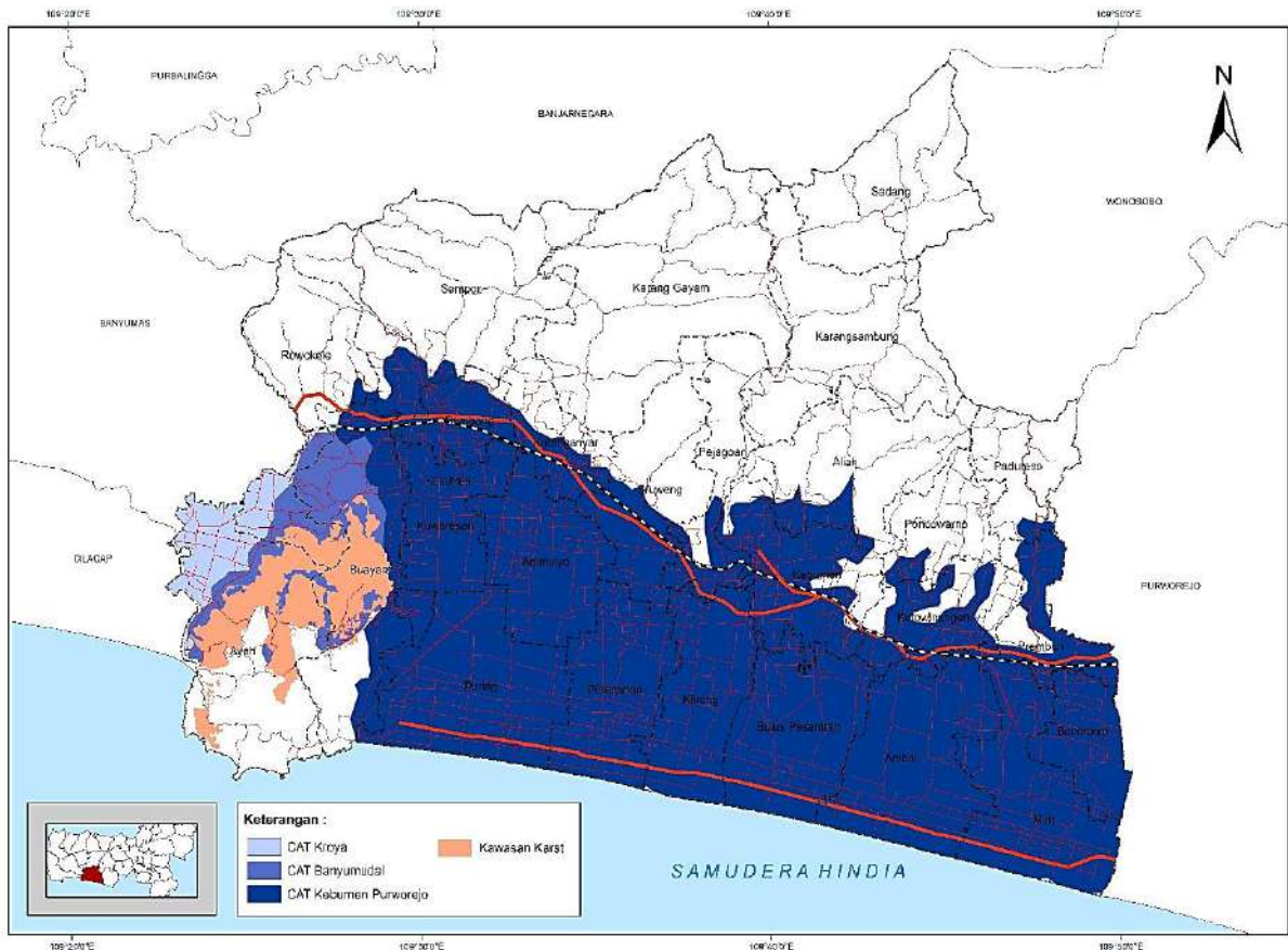
Gambar 2.3 Peta Hidrogeologi Kabupaten Kebumen
